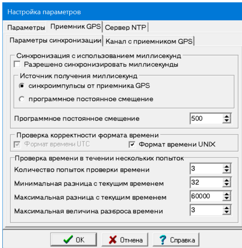
Центр синхронизации времени. Настройка параметров приемника GPS
