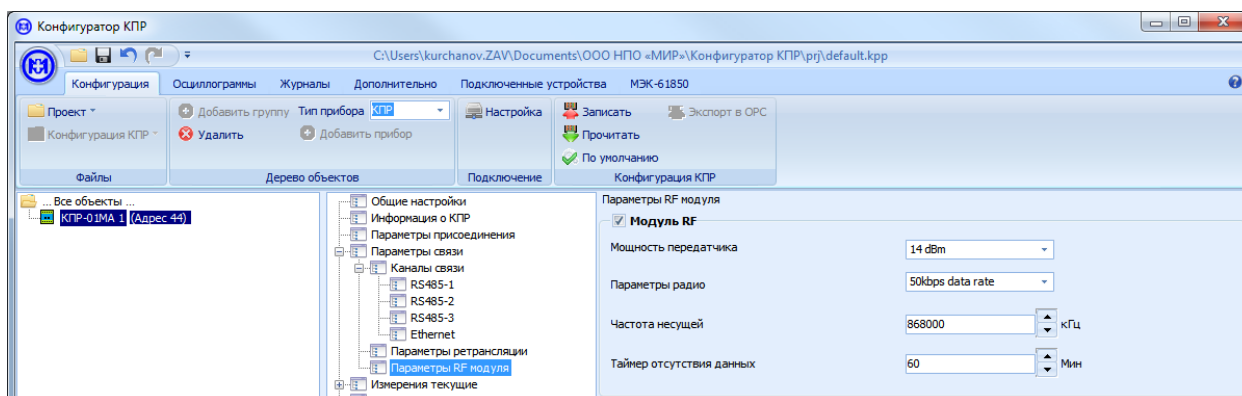
Рисунок 6.12 – Параметры RF модуля
