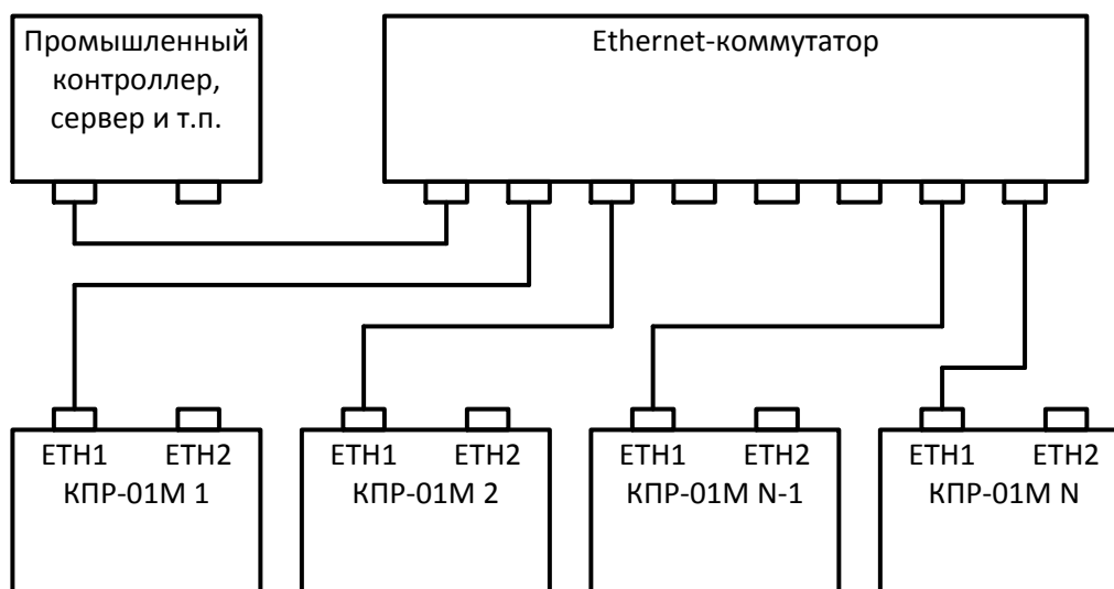
Рисунок 5.4 – Радиальная схема подключения к сети Ethernet
