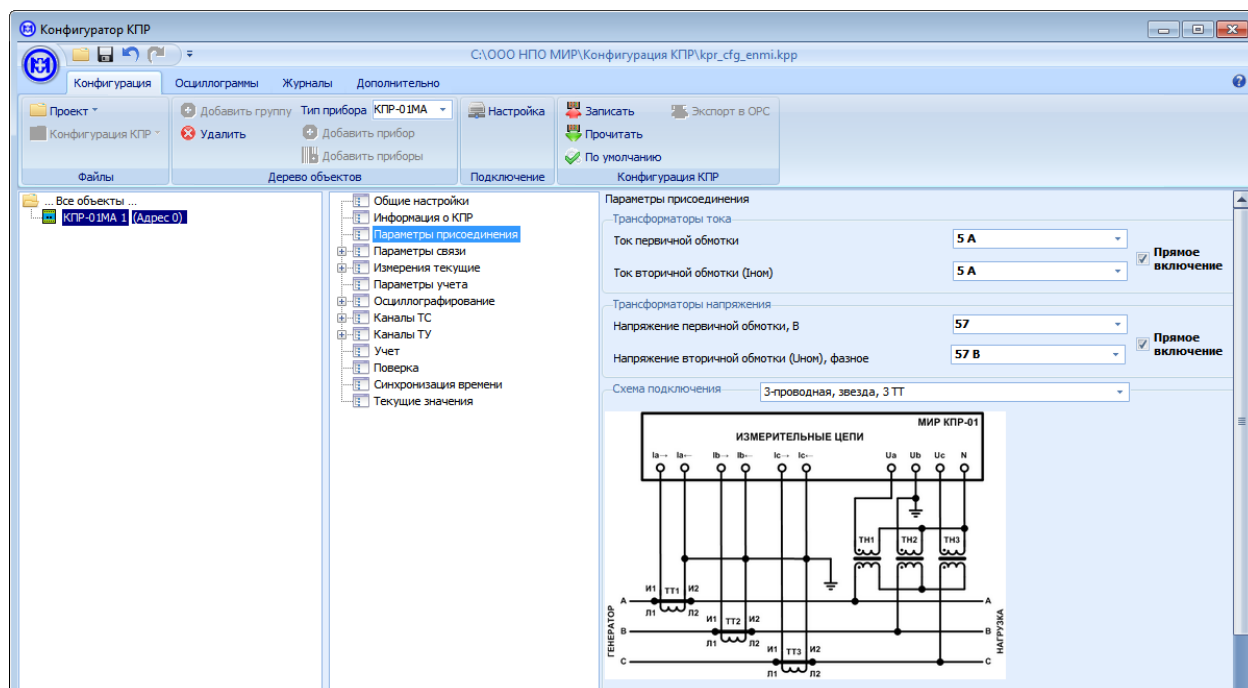
Рисунок 6.9 – Параметры присоединения
