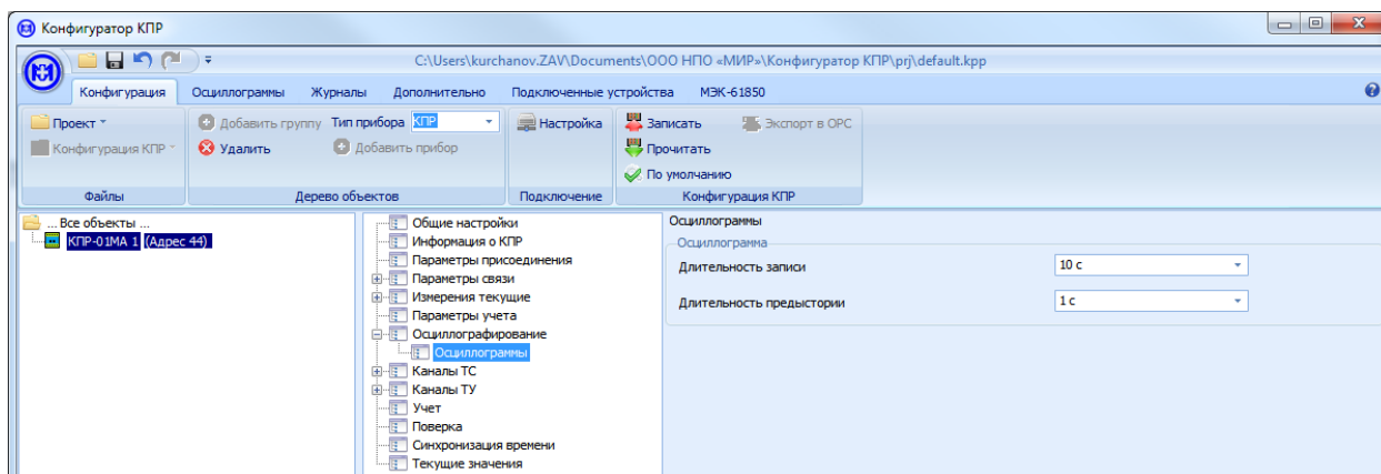
Рисунок 6.19 – Параметры осциллограммы
