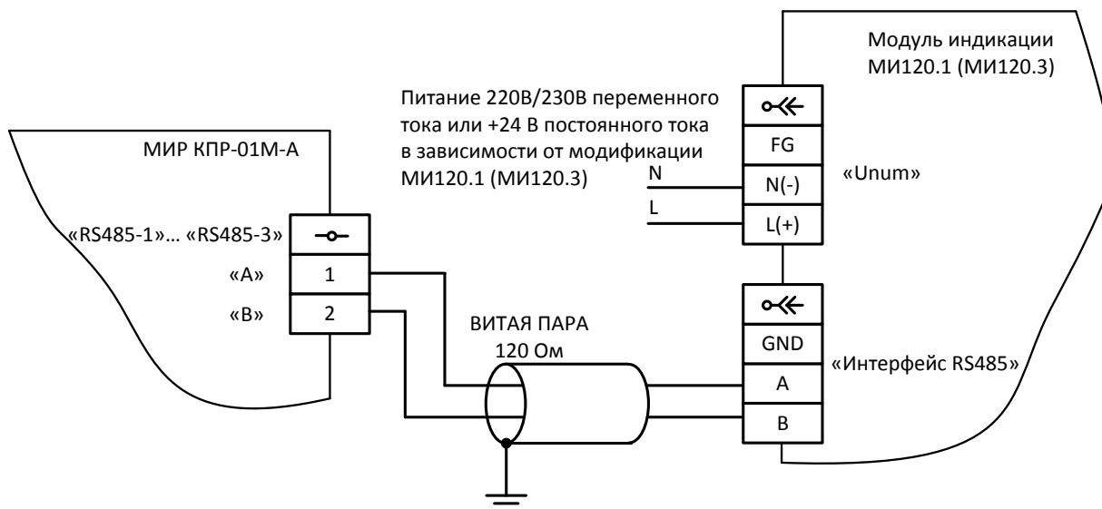
Рисунок 5.7 – Схема подключения внешних модулей индикации МИ120.1 и МИ120.3
