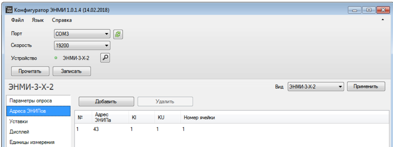
Рисунок 5.10 – Параметры активного режима работы ЭНМИ-3 (задание адреса)
