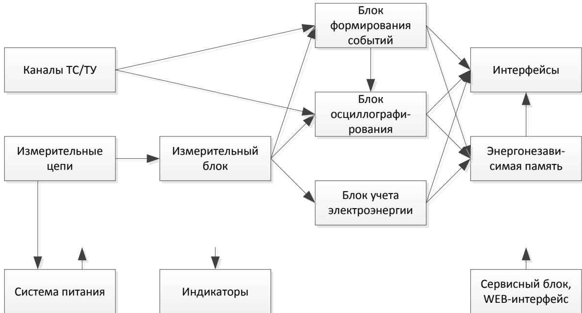
Рисунок 4.1 – Структурная схема изделия
