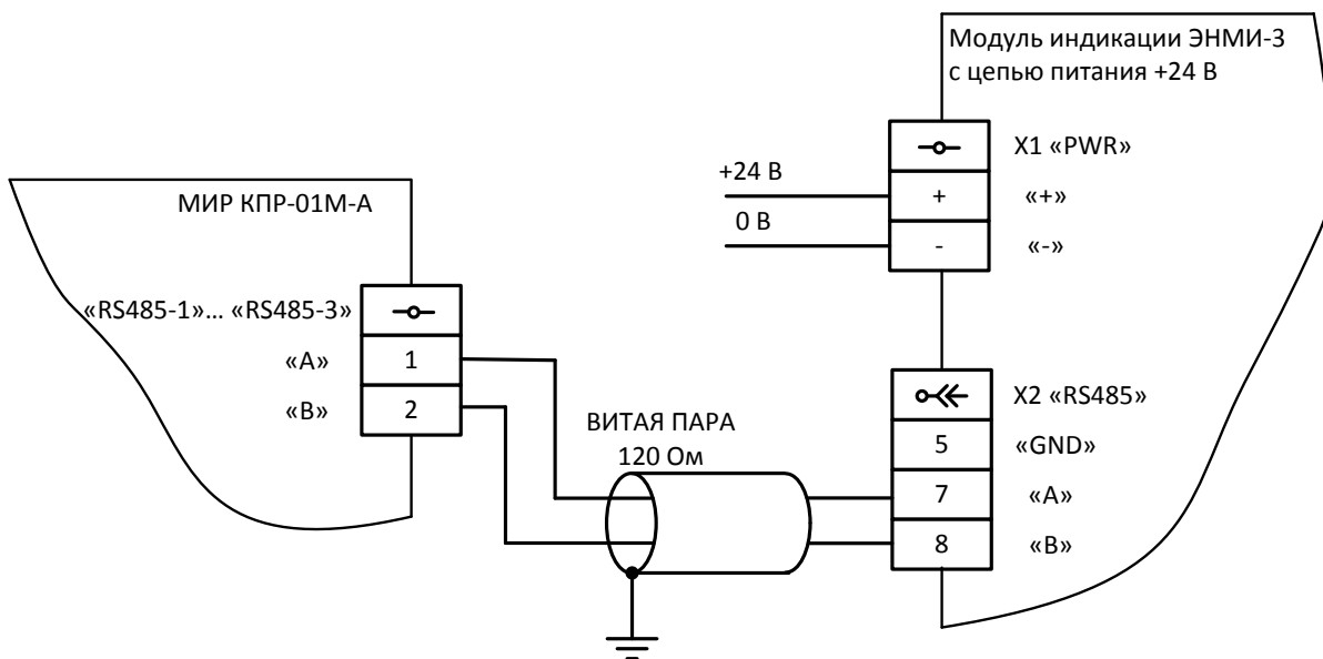
Рисунок 5.6 – Схема подключения внешнего модуля индикации ЭНМИ-3
